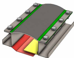
Convogliatore flottante
